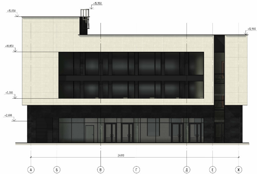
Фасад А-Ж
